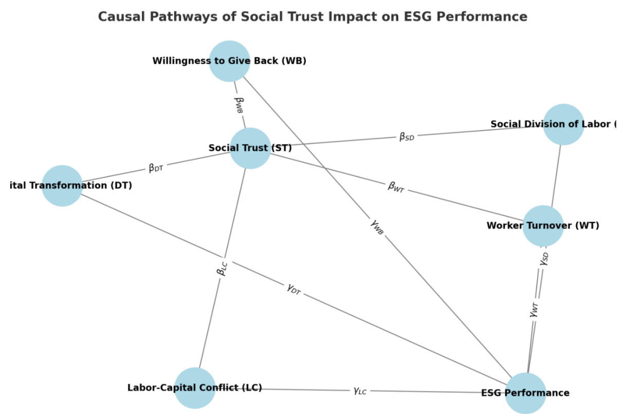
图 3：因果路径图
