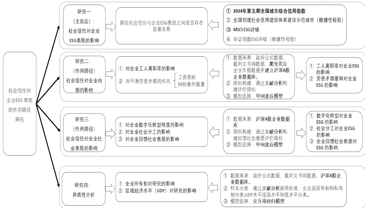
图 2：研究思路图
